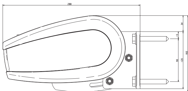
Väggmontering
